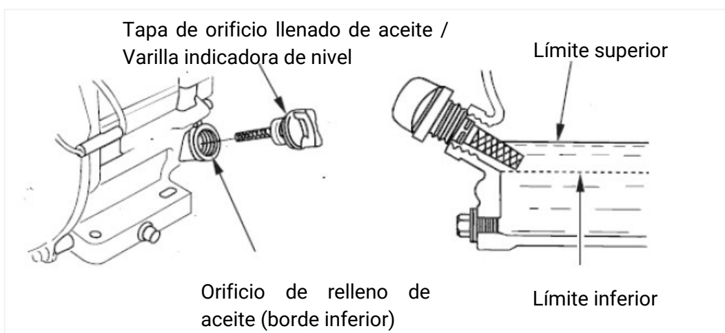
Imagen 9: Esquema componentes comprobación nivel de aceite.
