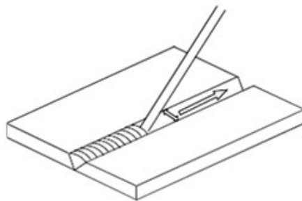
Imagen 15: Esquema buenas prácticas de soldadura con electrodo.
