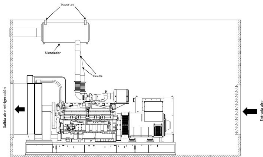
Disposición típica de Grupo Electrógeno en sala cerrada
