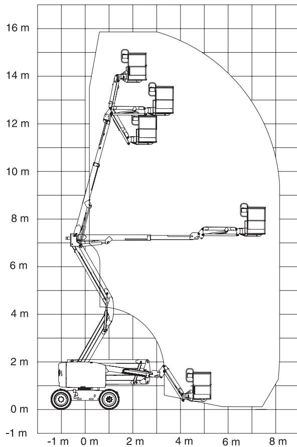
Diagrama de radios de acción de los modelos Z-45/25J
