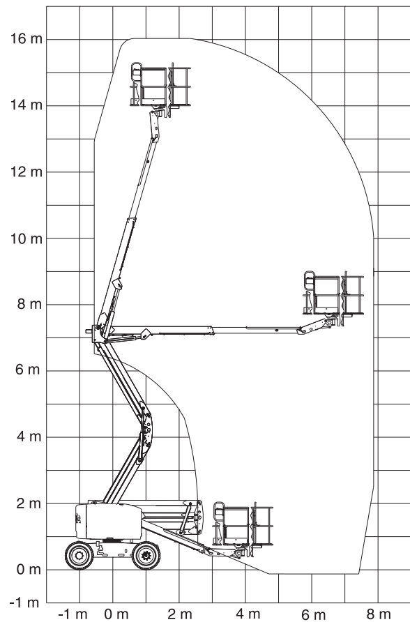
Diagrama de radios de acción de los modelos Z-45/25
