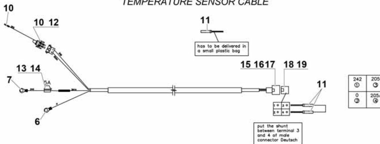
CÂBLE CAPTEUR TEMPERATURE/ TEMPERATURE SENSOR CABLE
