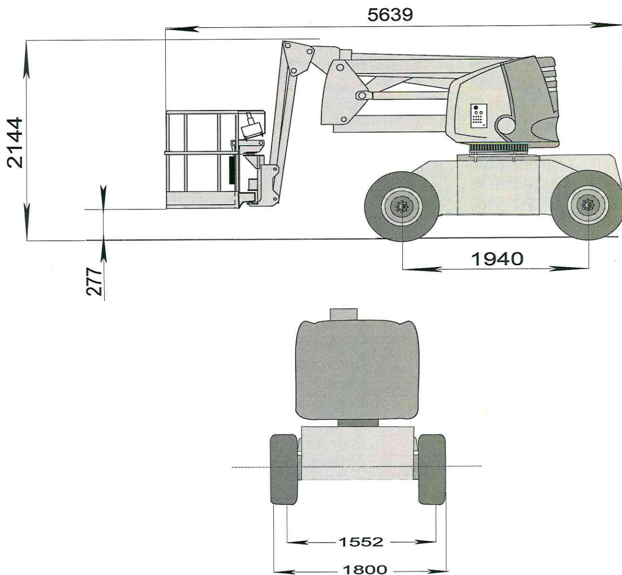
Fig. 4 - Dimensiones
